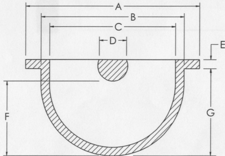
SECTION A-A SCALE 5:3
